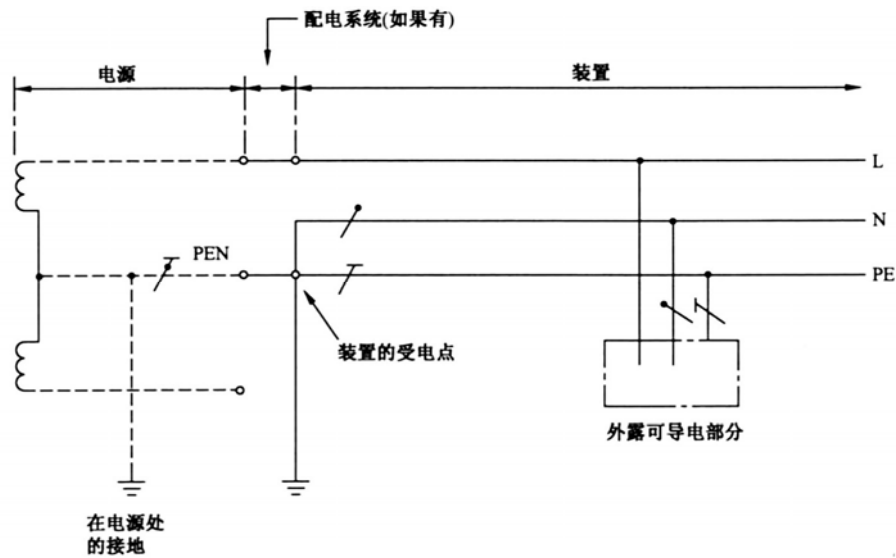
图 7.1.1-6 在装置的受电点将 PEN 分离成 PE 和 N 的单相 2 线制的 TN-C-S 系统
