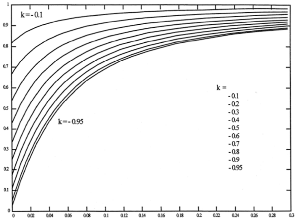
图 C.0.1 C_s 受 h 和 K 变化的曲线
