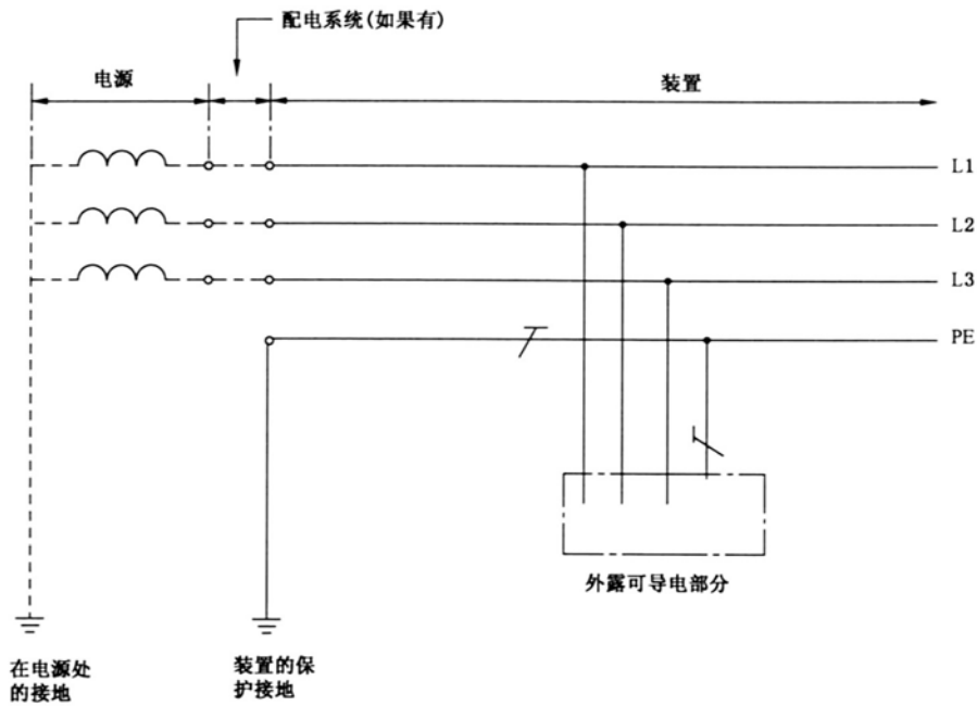
图 7.1.2-2 全部装置都具有接地的保护导体，但不配出中性导体的 TT 系统
